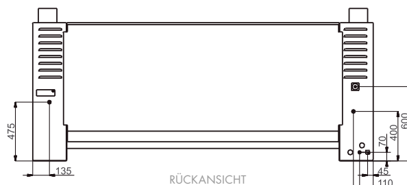
RÜCKANSICHT
